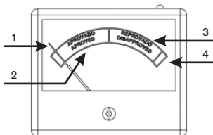
Figura 3 - Painel do galvanômetro
